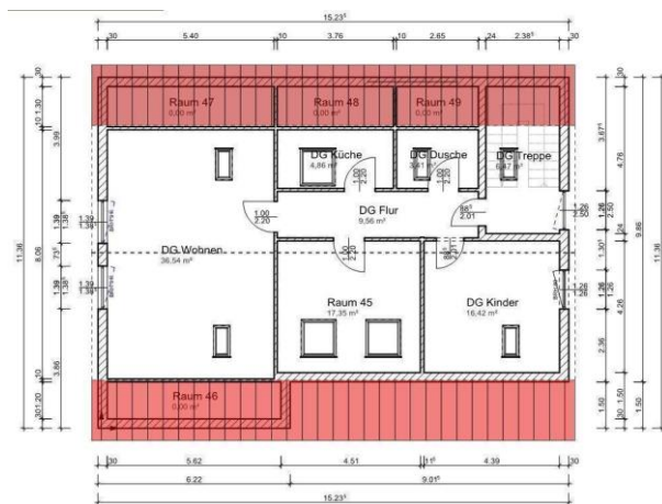
Grundriss Dachgeschoss
